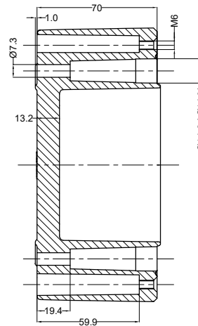
SECTION D-D
