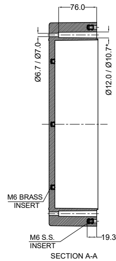
SECTION A-A
