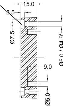
SECTION A-A
