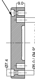
SECTION A-A
