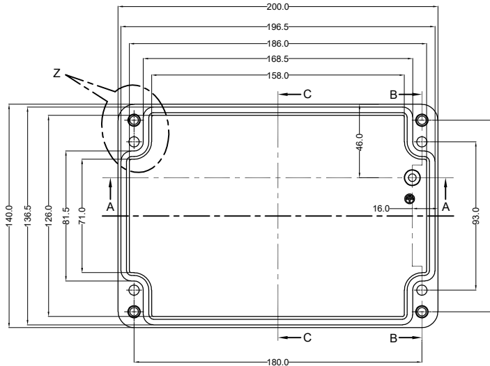
LID
