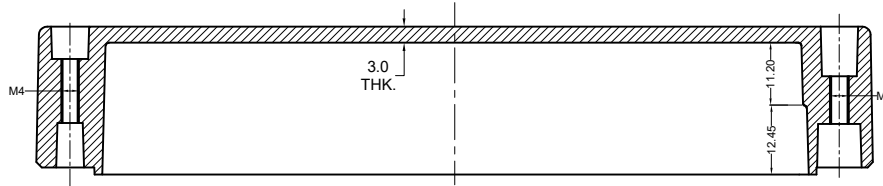
SECTION D-D
